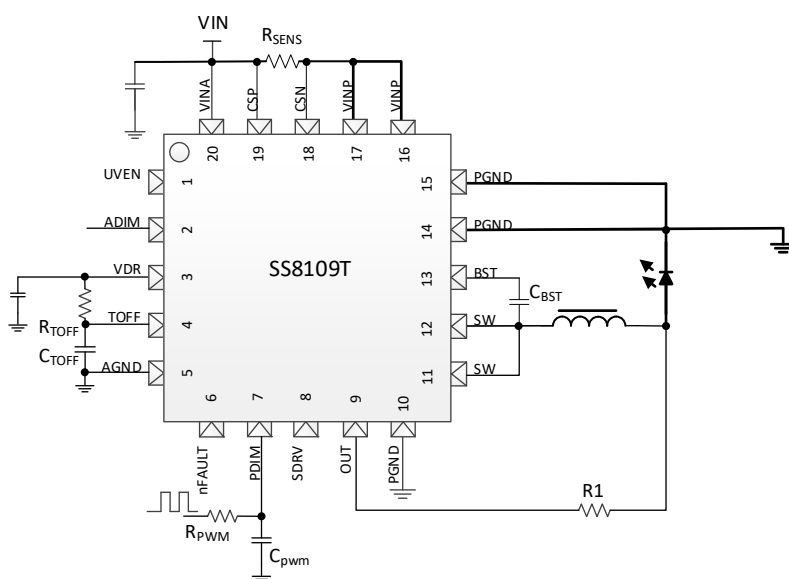
图 1 应用原理图（通用调光模式）
