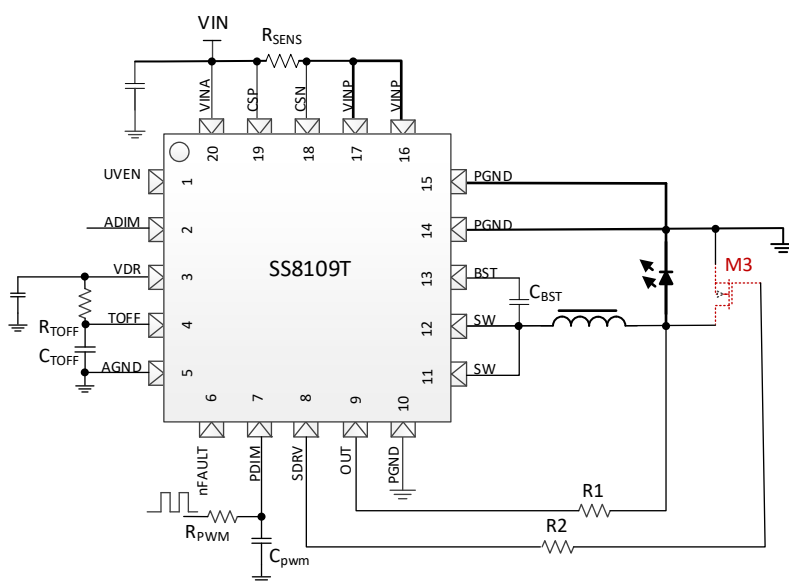
图 2 应用原理图（并联调光模式）
